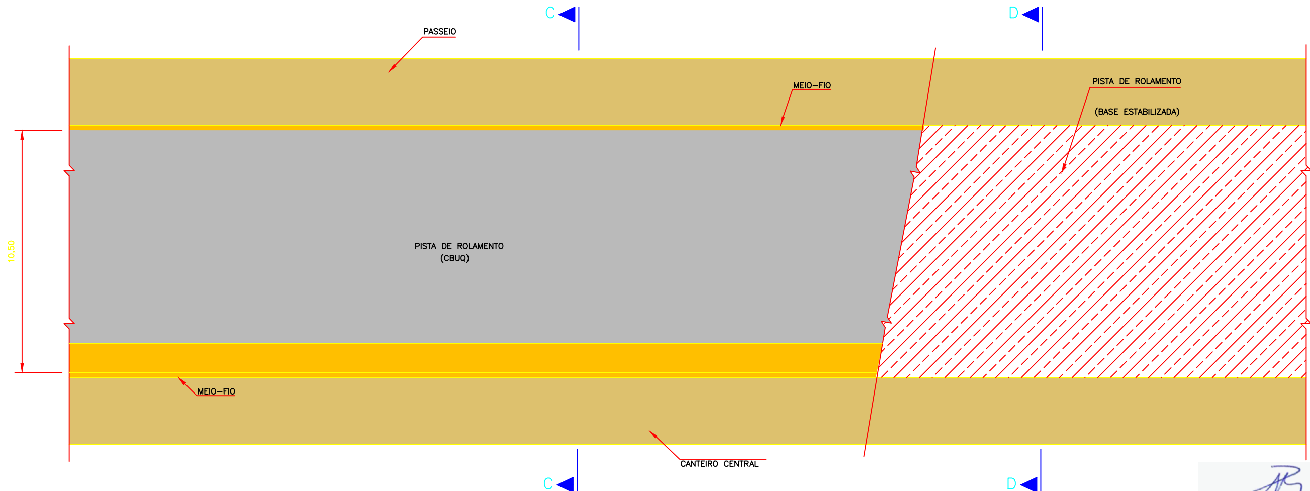
PAVIMENTAÇÃO TÍPICA - 02 PLANTA ESC. 1:100
